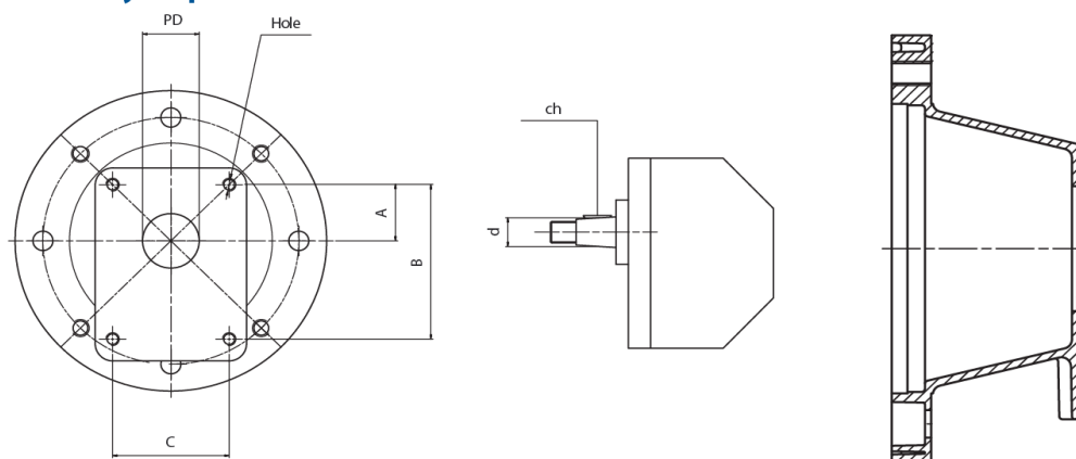
Parametry čerpadel
