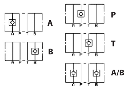
Hydraulické schéma
